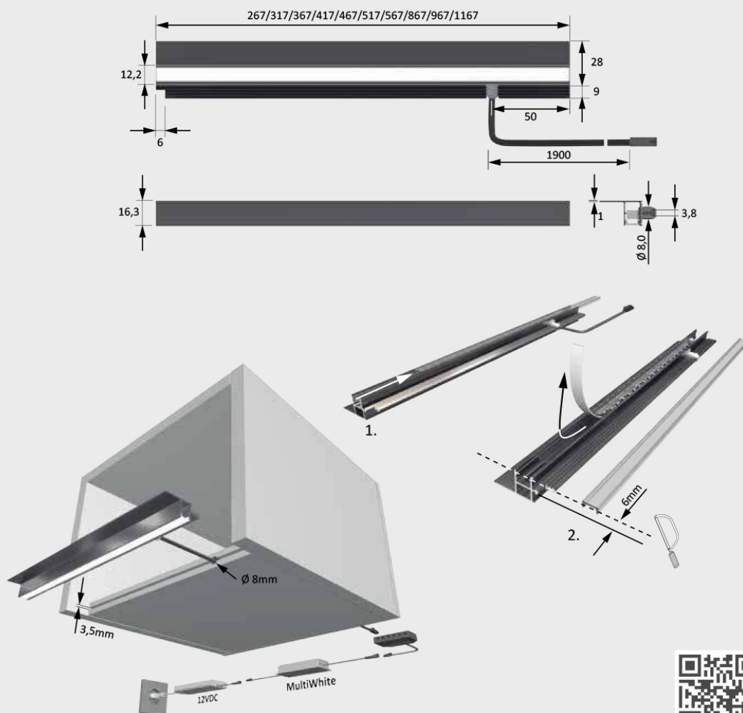
Esquema de montaje
